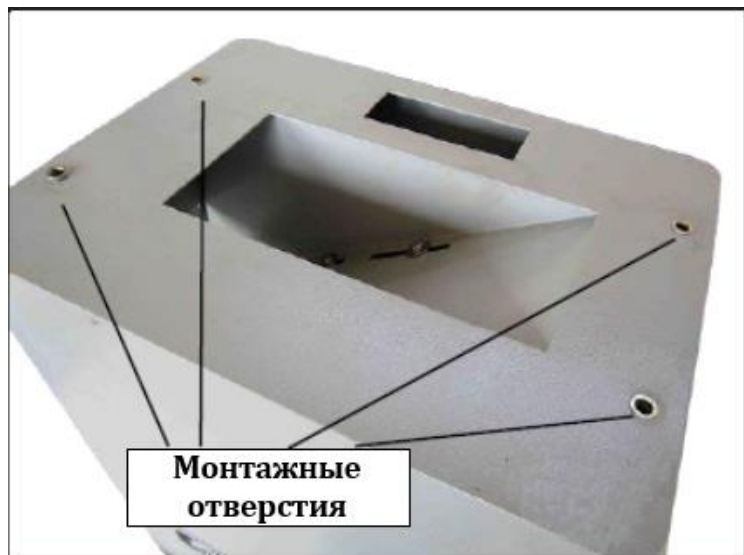
Рис. 3. Монтажные отверстия
